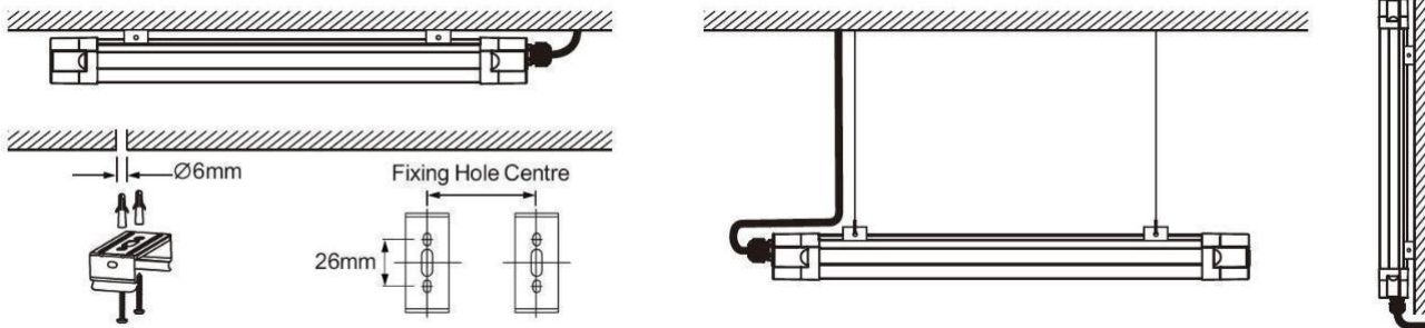
Formas de montaje
